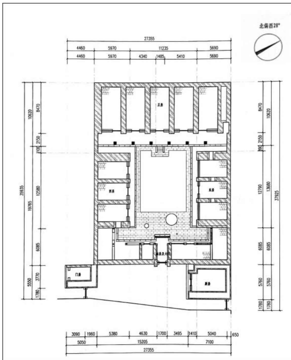
中央后委机关旧址—粮草院旧址平面示意图
