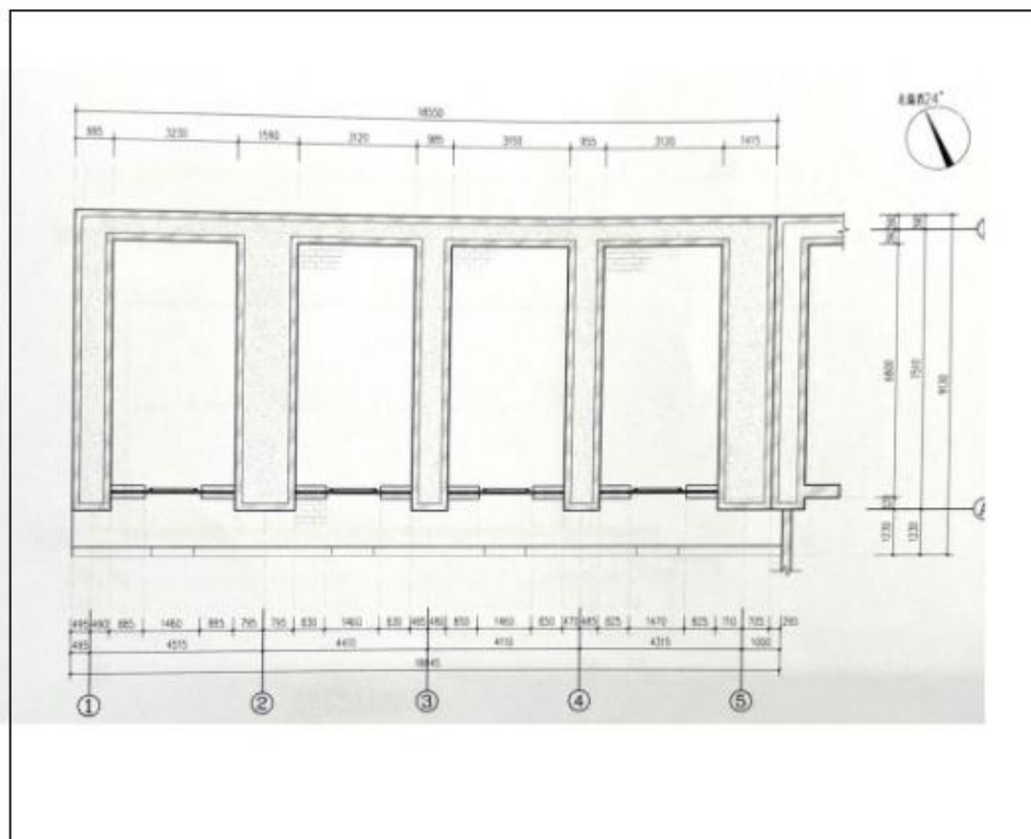
中央后委机关旧址—叶剑英同志旧居平面示意图
