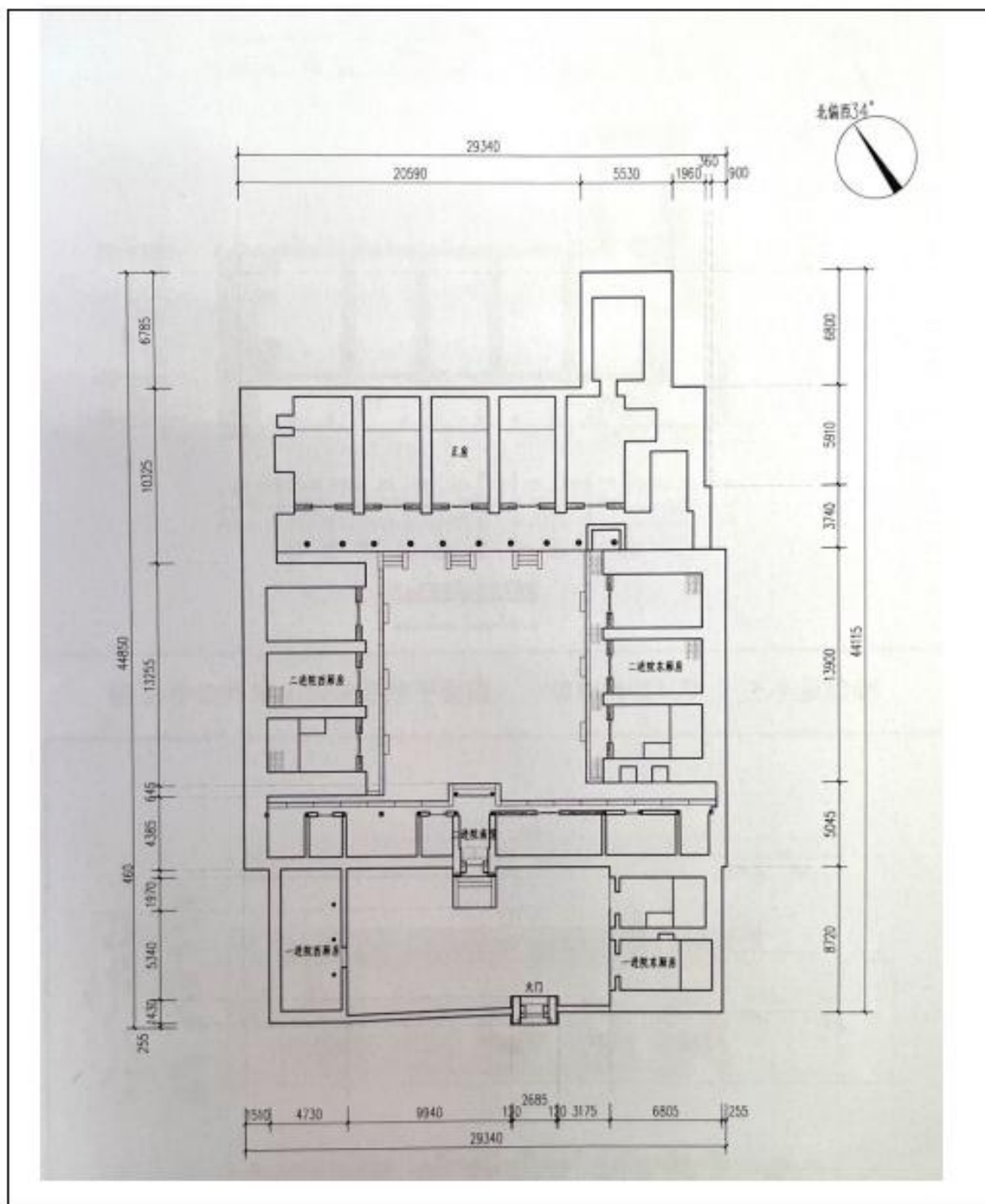
中央后委机关旧址—中央外事组旧址平面示意图
