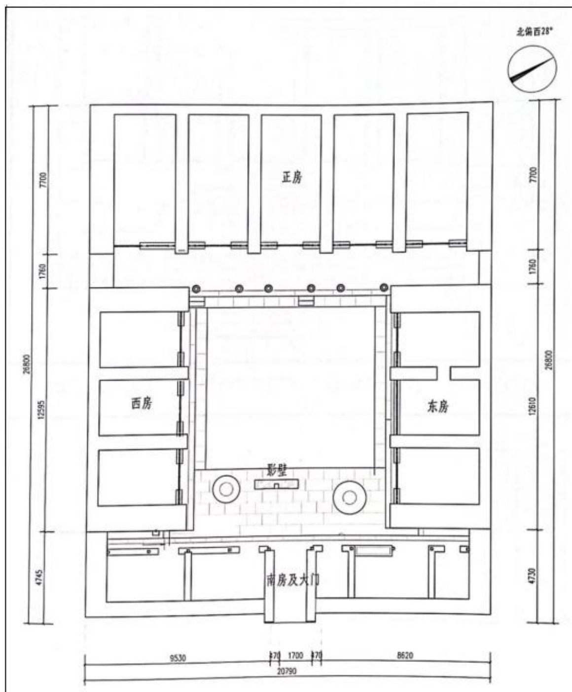
中央后委机关旧址—杨尚昆旧居平面示意图
