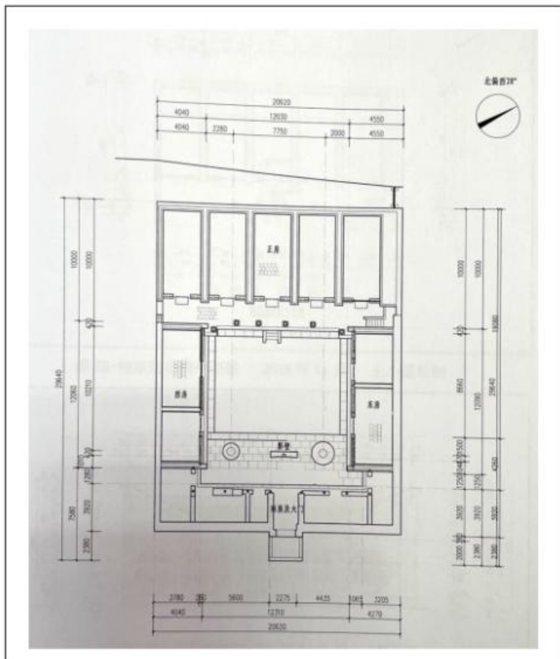
中央后委机关旧址—军委作战部旧址平面示意图
