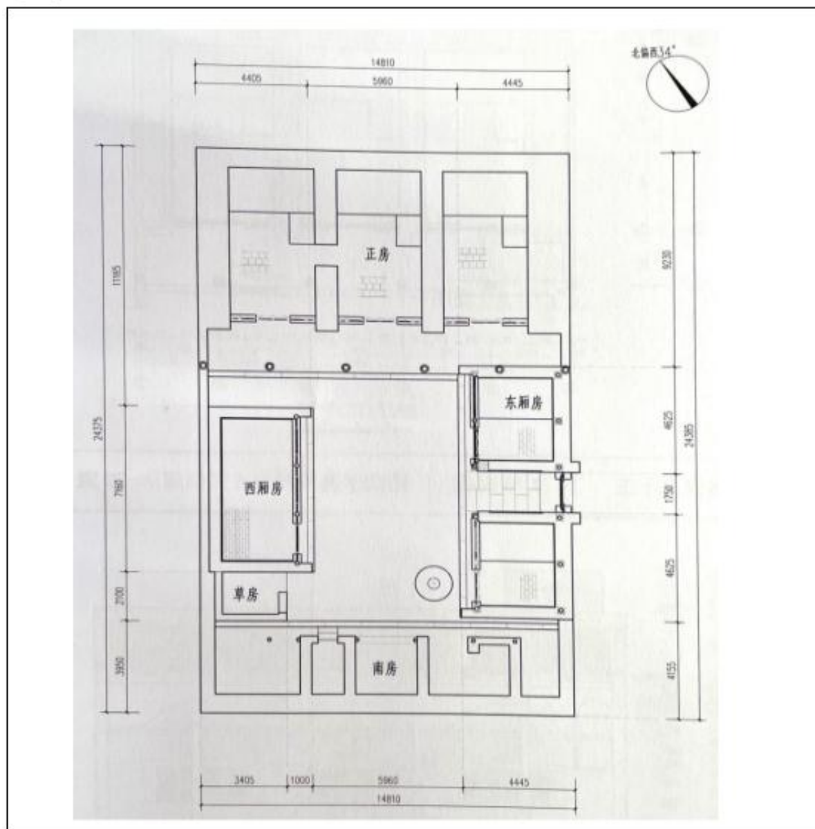
中央后委机关旧址—中央书记处特别会计室旧址平面示意图
